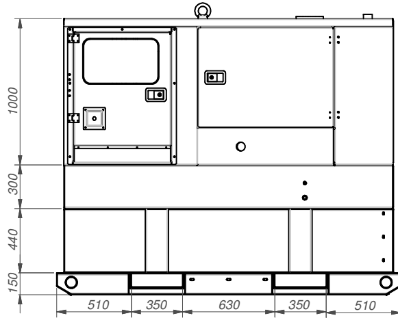
GRUPO ELECTRÓGENO CON BANDEJA DE RETENCIÓN 48h. (725 L) Y PATINES GALVANIZADOS OPTIONAL 48h. FUEL TANK AND RETENTION BATH (725 L) AND ZINCCOATED SKIDS
