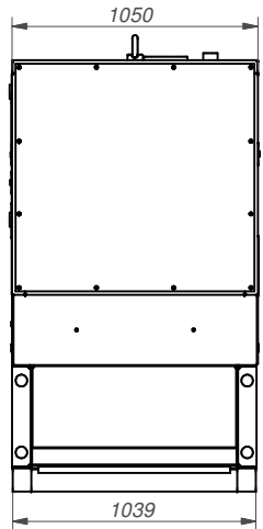
GRUPO ELECTRÓGENO CON BANEJA DE RETENCIÓN 48h. (725 L) CON PATAS DE SOPORTE OPTIONAL 48h. FUEL TANK AND RETENTION BATH (725 L) WITH SUPPORTS
