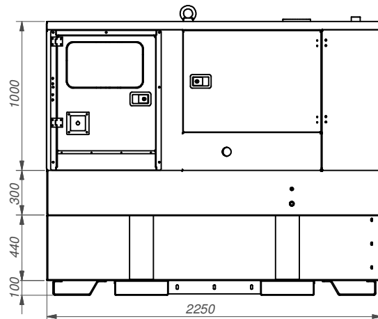
GRUPO ELECTRÓGENO CON BANEJA DE RETENCIÓN 48h. (725 L) CON PATAS DE SOPORTE OPTIONAL 48h. FUEL TANK AND RETENTION BATH (725 L) WITH SUPPORTS
