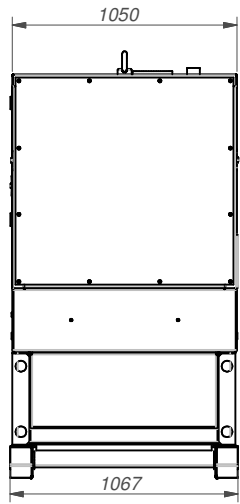
GRUPO ELECTRÓGENO CON BANDEJA DE RETENCIÓN 48h. (725 L) Y PATINES GALVANIZADOS OPTIONAL 48h. FUEL TANK AND RETENTION BATH (725 L) AND ZINCCOATED SKIDS
